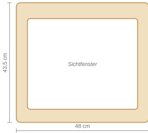
Vorderrahmen mit Sichtfenster (48 x 43,5 cm)
